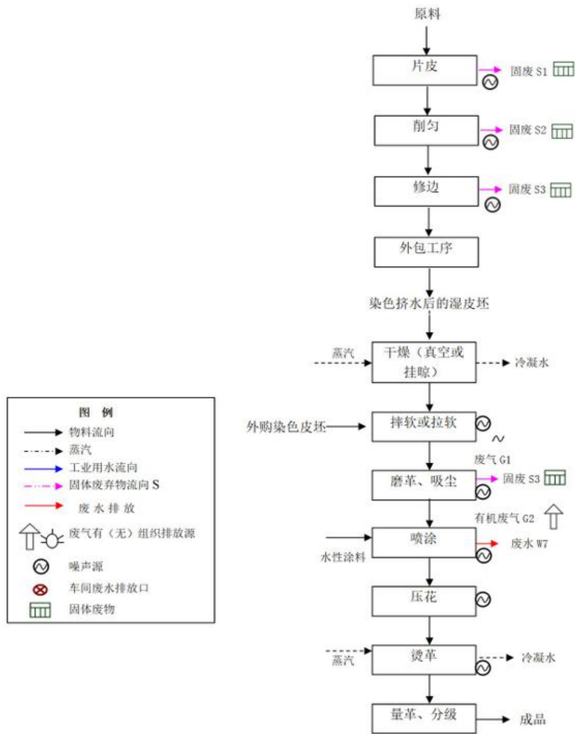
图5.1-1 生产工艺流程及产污环节图
